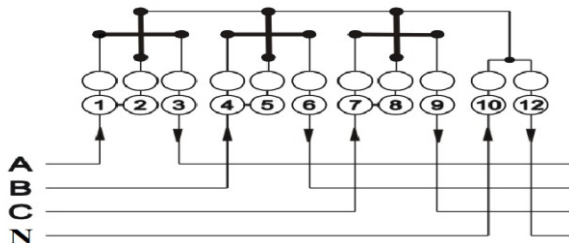
Sơ đồ đấu dây mạch 3 pha 4 dây trực tiếp 3 phase 4 wire direct connection diagrams
