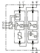
Prinzipschaltbild DG MP TT 2P ACI 275 FM
